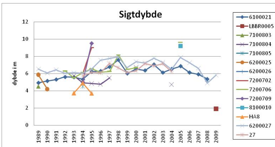
Figur 3. Den gennemsnitlige sigtddybde i Lillebælt fra 1989-2009. Sigtddybden har på størstedelen af stationerne ligget omkring 6 meter indtil midten af 1990'erne, mellem 6 og 8 meter indtil 2006, hvorefter antallet af målestationer er faldet. Fra midt 1990'erne og indtil midt 2000'erne har sigtddybden ligget mellem 6-8 meter, hvorefter den er faldet til under 6 meter. Placeringen af de enkelte stationer ses på Figur 1.
