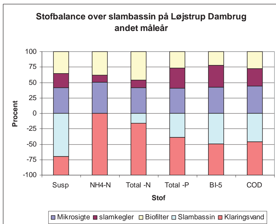
Figur 27 Kilder til stoftilførsel og stoffjernelse over slambassinet på Løjstrup Dambrug (øst) det andet måleår. Stofinput til slambassinene kommer fra returskylling af biofiltere, tømning af slamkegler samt spulevand fra mikrosigterne. Stofindholdet i klaringsvandet er udtryk for den stofmængde, der tabes fra slambassin til plantelagune.
