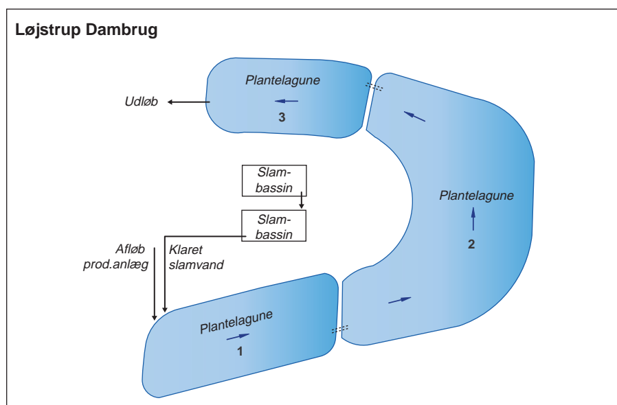
Figur 29 Principskitse af plantelagunen på Løjstrup Dambrug (øst) med de tre søagtige bassiner. Se også figur 1 i kapitel 2.
