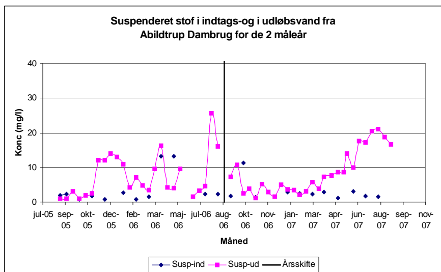
Figur 27 Suspenderet stof koncentrationen (mg/l) i indtagstvandet til Abildtrup Dambrug og i afløbet til Vorgod Å i første og andet måleår.
