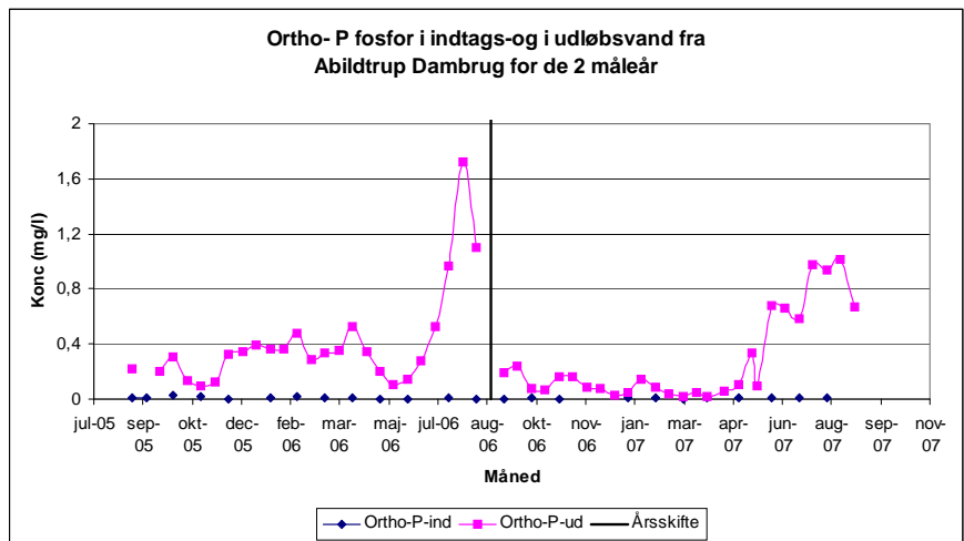
Figur 23 Orthofosfat fosfor koncentrationen (mg/l) i indtagsvandet til Abildtrup Dambrug og i udløbet fra dambruget til Vorgod Å i første og andet måleår.
