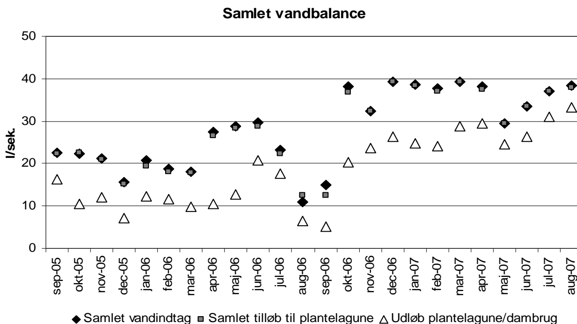
Figur 9 Samlet vandbalance (l/s) over Abildtrup Dambruget, månedsmiddel.
