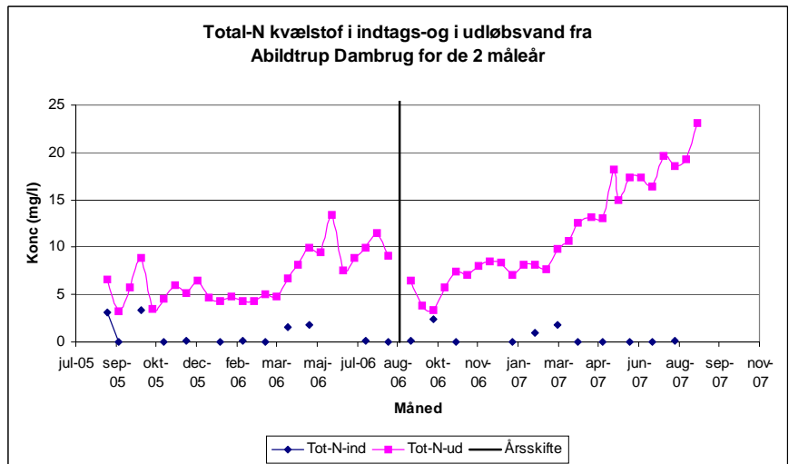
Figur 22 Total kvælstof koncentrationen (mg/l) i indtagsvandet til Abildtrup Dambrug og i udløbet fra dambruget til Vorgod Å i første og andet måleår.
