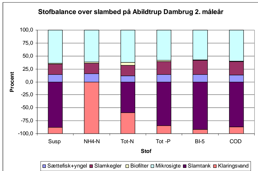
Figur 28 Kilder til stoftilførsel og stoffjernelse over slamtank på Abildtrup Dambrug i andet måleår. Stofinputtet kommer fra returskyllning af biofiltere, tømning af slamkegler samt spulevand fra mikrosigterne. Stoffindholdet i klaringsvandet er udtryk for den stofmængde, der tabes fra slamtank til plantelagune.
