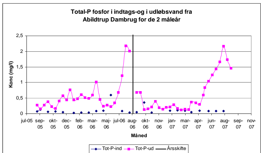
Figur 24 Total fosfor koncentrationen (mg/l) i indtagsvandet til Abildtrup Dambrug og i udløbet herfra til Vorgod Å i første og andet måleår.
