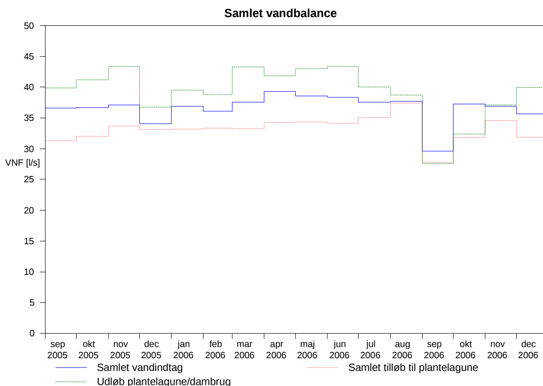
Figur 5 Samlet vandbalance over Tingkærvad Dambrug, månedsmiddel (l/s)
