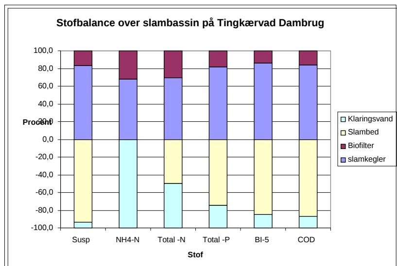
Figur 19 Stofbalance over slambassin på Tingkærvad Dambrug. Input til slambassin er beregnet som summen af de enkelte bidrag fra skylning af biofiltre og slamkegler. Det samlede input til slambassin er sat til 100 % og er angivet som positive værdier. Tilsvarende er summen af tilbageholdelsen og fraførelsen (klaringsvandet til plantelagunen) sat til 100 % på negativsiden af skalaen. Tilbageholdelsen i slambassin er beregnet som summen af input til slambassin minus fraførelsen med klaringsvandet. Ammonium bliver produceret i slambassin og der føres i virkeligheden 160 % bort sammenlignet med tilførslen af ammonium-kvælstof med klaringsvandet, men af grafiske årsager er den sat til -100 %.
