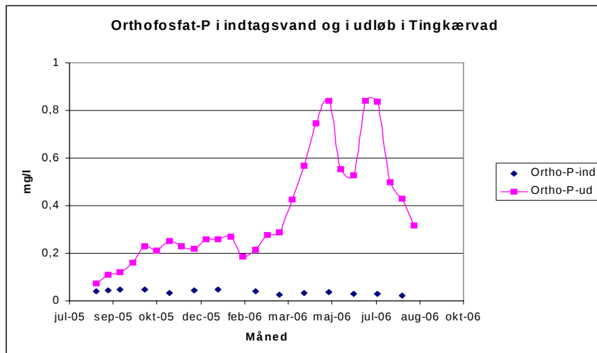
Figur 12 Orthofosfat-fosfor koncentrationen (mg/l) i indtagstvåndet og i udløbet til Vejle Å i det første måleår på Tingkærvad Dambrug.
