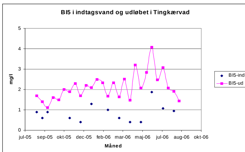
Figur 14 Organisk stof målt som BI 5 koncentrationen (mg/l) i indtagstvåndet og i udløbet til Vejle Å i det første måleår på Tingkærvad Dambrug.
