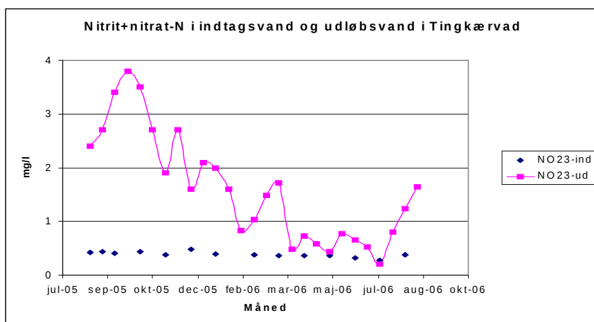
Figur 10 Nitrit+Nitrat-kvælstof koncentrationen (mg/l) i indtagstvånd og i udløbet til Vejle Å i det første måleår på Tingkærvad Dambrug.
