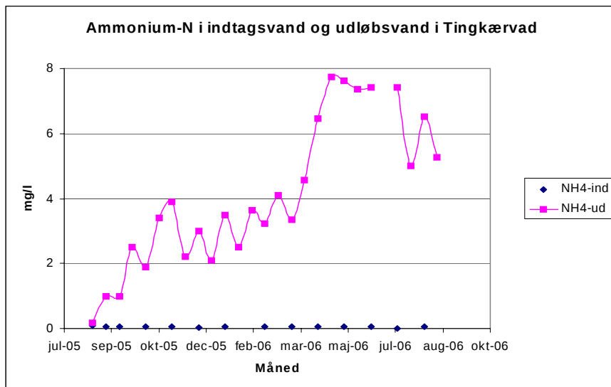
Figur 9 Ammonium-kvælstof koncentrationen (mg/l) i indtagstvåndet og i udløbet til Vejle Å i det første måleår på Tingkærvad Dambrug.
