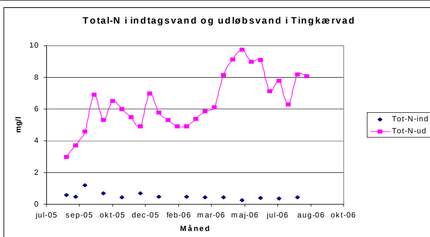
Figur 11 Total-kvælstof koncentrationen (mg/l) i indtagstvåndet og i udløbet til Vejle Å i det første måleår på Tingkærvad Dambrug.
