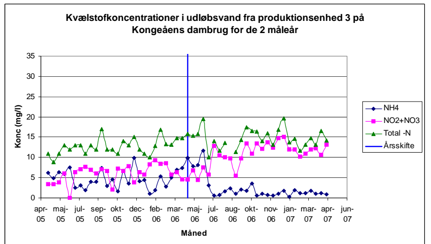
Figur 13-15 Koncentrationsudvikling i de tre produktionsenheder (nr. 1 figur 13, nr. 2 figur 14 og nr. 3 figur 15) på Kongeåens Dambrug over de to måleår for ammonium-N, nitrit+nitrat-N samt total-N nedstrøms biofiltre svarende til koncentrationerne i det vand, der løber ind i plantelagunen fra produktionsenhederne.
