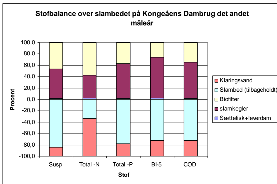
Figur 33 Stoffjernelse over slambassinene på Kongeåens Dambrug det andet måleår. Stoffinput til slambassinene tilføres fra returskylning af biofiltre og tømning af slamkegler i det samlede produktionsanlæg inkl. sættefisk + leveredam. Stoffindholdet i klaringsvandet er udtryk for den stofmængde, der tabes fra slambassinene.
