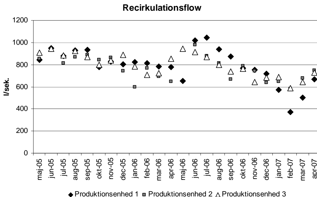
Figur 12 Recirkulationsflow i Kongeåens 3 produktionsenheder over de to måleår, månedsmiddel, l/s.
