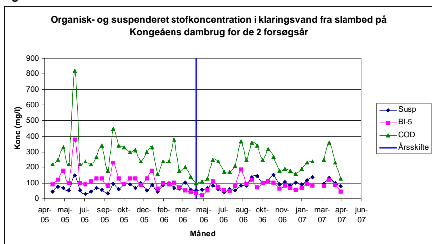
Figur 22-24 Koncentrationen af kvælstoffraktioner (ammonium-N, nitrit+nitrat-N, total-N), fosforfraktioner (ortho-P, total-P), organisk stof (BI5, COD) samt suspenderet stof i klaringsvand fra slambassiner. Klaringsvandet løber til plantelagunen.
