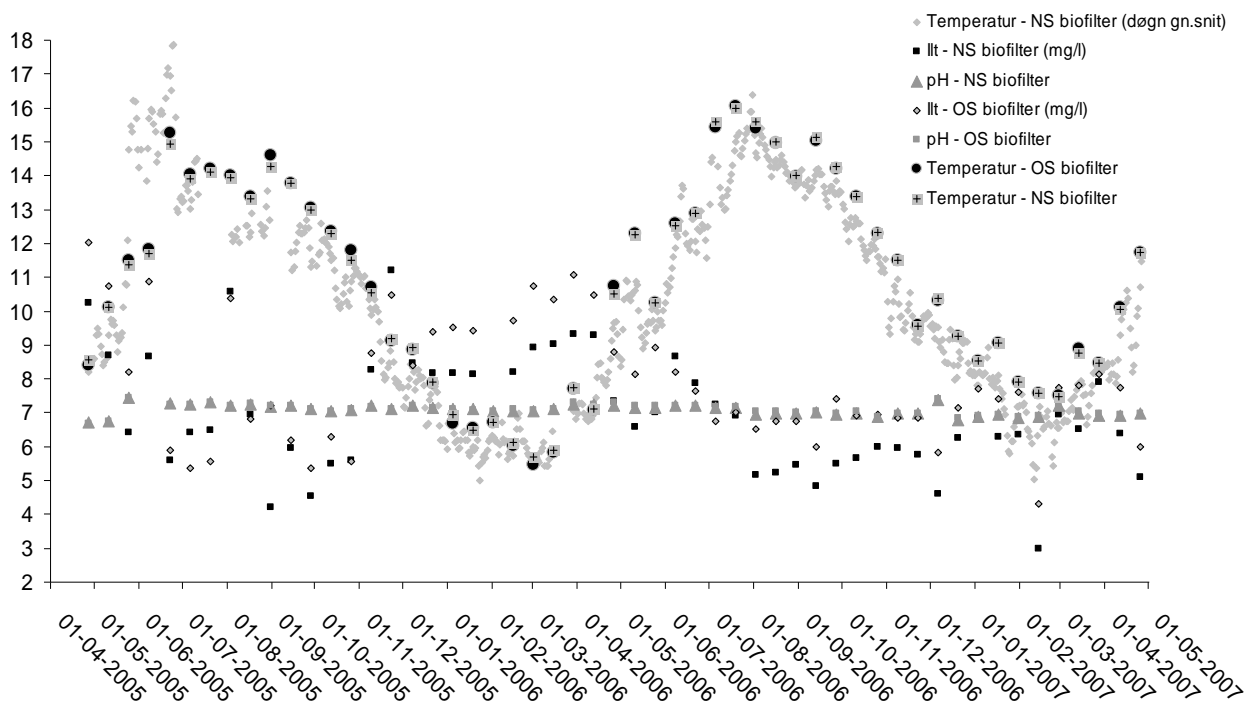
Figur 4 Ilt (mg/l), pH og temperatur (° C) angivet som gennemsnitsværdier for de tre produktionsenheder på Kongeåens Dambrug over begge måleår.
