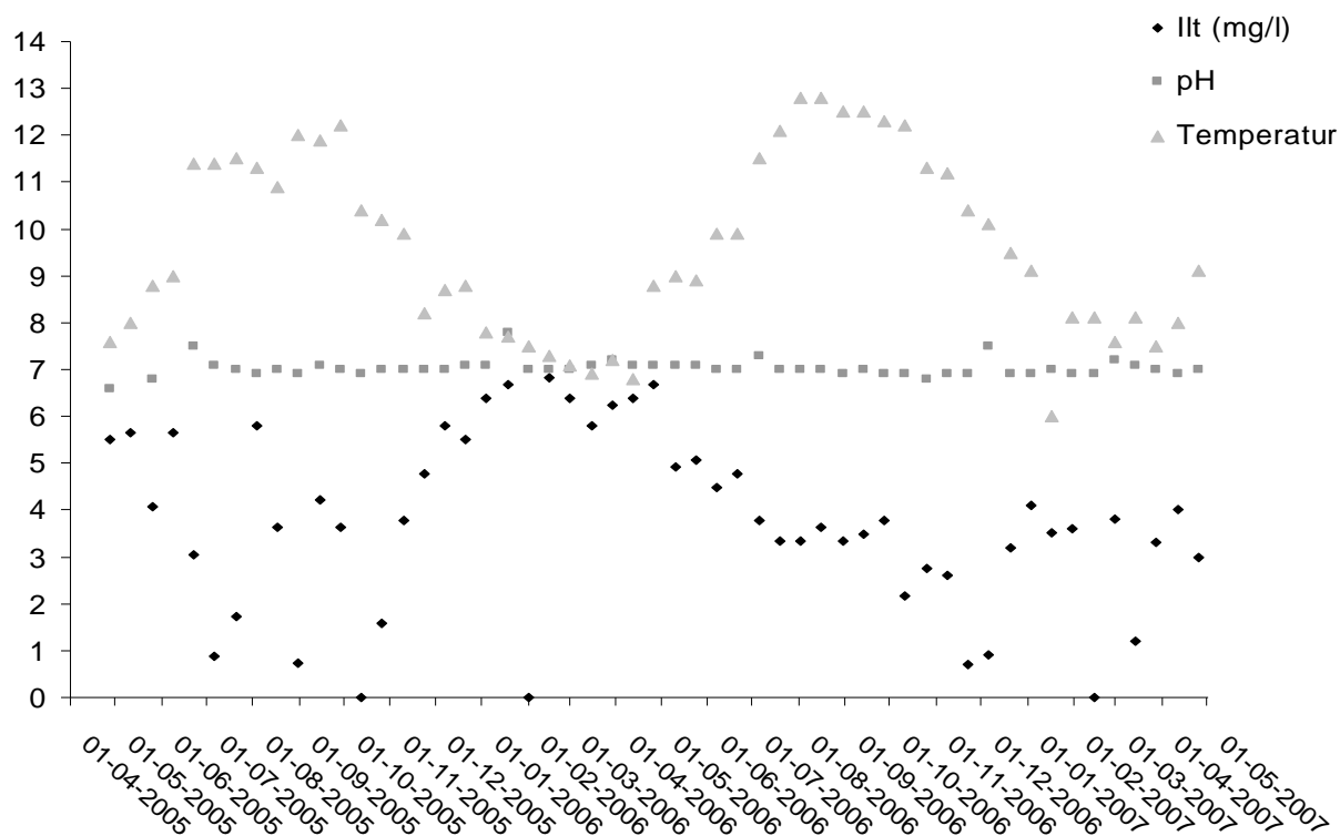
Figur 3 (mg/l), pH og temperatur (°C) målt hver 14. dag i indløbsvandet til produktionen på Kongeåens Dambrug over de to målear.
