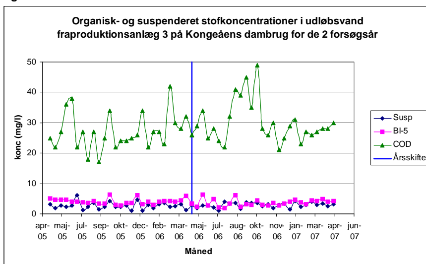
Figur 19-21 Koncentrationsudvikling i de tre produktionsenheder (nr. 1 figur 19, nr. 2 figur 20 og nr. 3 figur 21) på Kongeåens Dambrug over de to måleår for organisk stof målt som BI5 og COD og suspenderet stof nedstrøms biofilter, svarende til koncentrationerne i det vand, der løber ind i plantelagunen fra produktionsenhederne.
