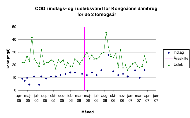
Figur 31 COD-koncentrationen (mg/l) i indtagsvandet til Kongeåens Dambrug og i afløbet fra dambruget til Kongeåen i første og andet måleår.
