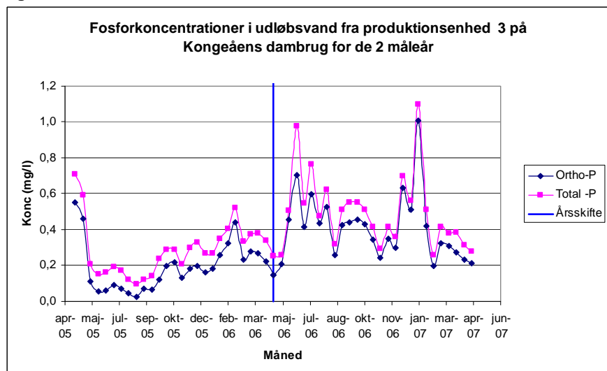
Figur 16-18 Koncentrationsudvikling i de tre produktionsenheder (nr. 1 figur 16, nr. 2 figur 17 og nr. 3 figur 18) på Kongeåens Dambrug over de to måleår for orthofosfat og total fosfor nedstrøms biofilter, svarende til koncentrationerne i det vand, der løber ind i plantelagunen fra produktionsenhederne.
