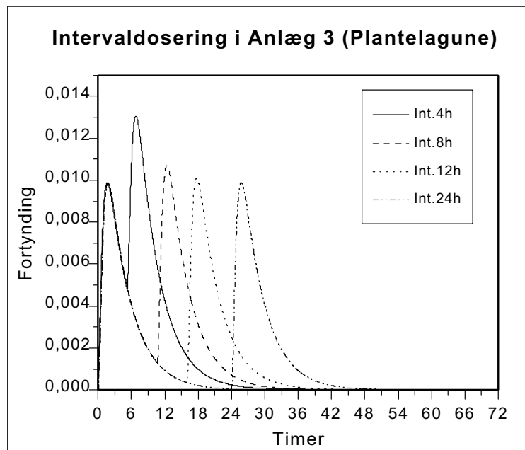
Figur 4.6 Koncentrationsforløb i plantelagunen i anlæg 3 af 2 på hinanden følgende doseringer henholdsvis 4, 8, 12 og 24 timer efter start
