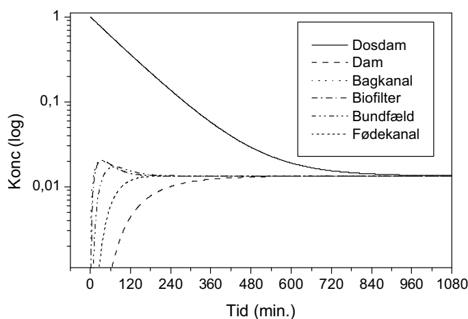
Konc. i dambrug ved 100 % recirkulering og dosering af 1 dam-3
