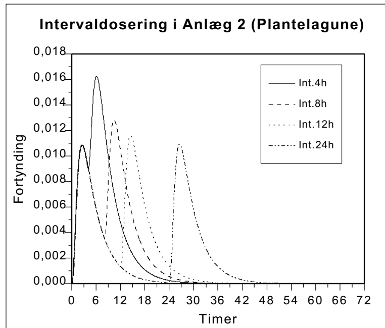
Figur 4.5 Koncentrationsforløb i plantelagunen i anlæg 2 af 2 på hinanden følgende doseringer henholdsvis 4, 8, 12 og 24 timer efter start
