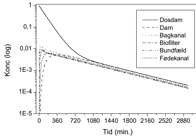
Konc i dambrug ved 100 % recirkulering og 30 % rensning i biofilter når 1 dam-2 er doseret
