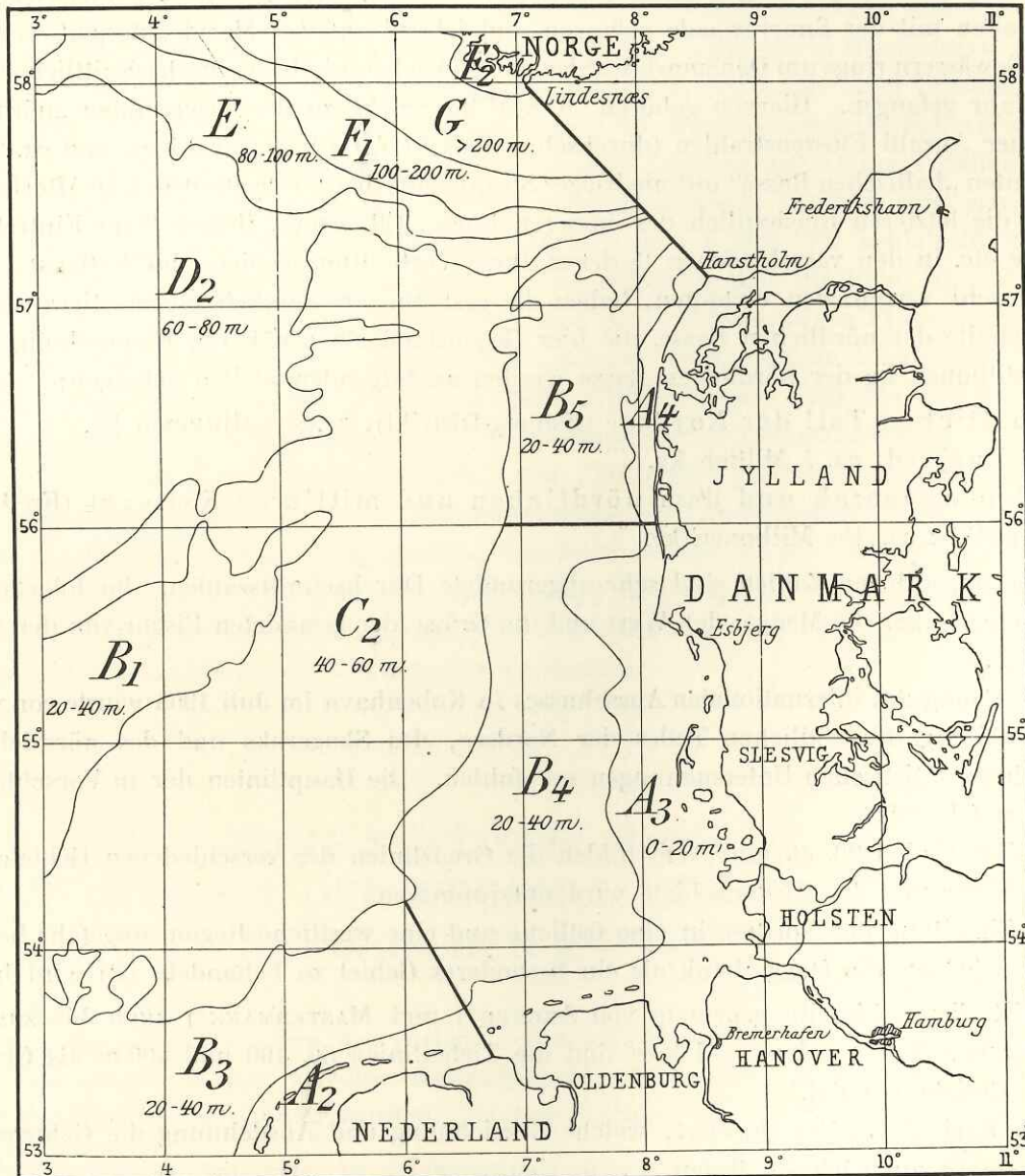
Fig. 1. Einteilung des östlichen Teiles der Nordsee nach Tiefenzonen.
