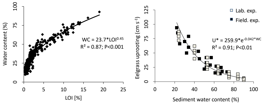
Figur B.2. Sammenhængen mellem LOI og Vandindhold (venstre) og forankrings-kapaciteten for ålegræs fra rent sand (20% vandindhold) til flydende mudder (90% vandindhold) målt i feltet og laboratoriet.
