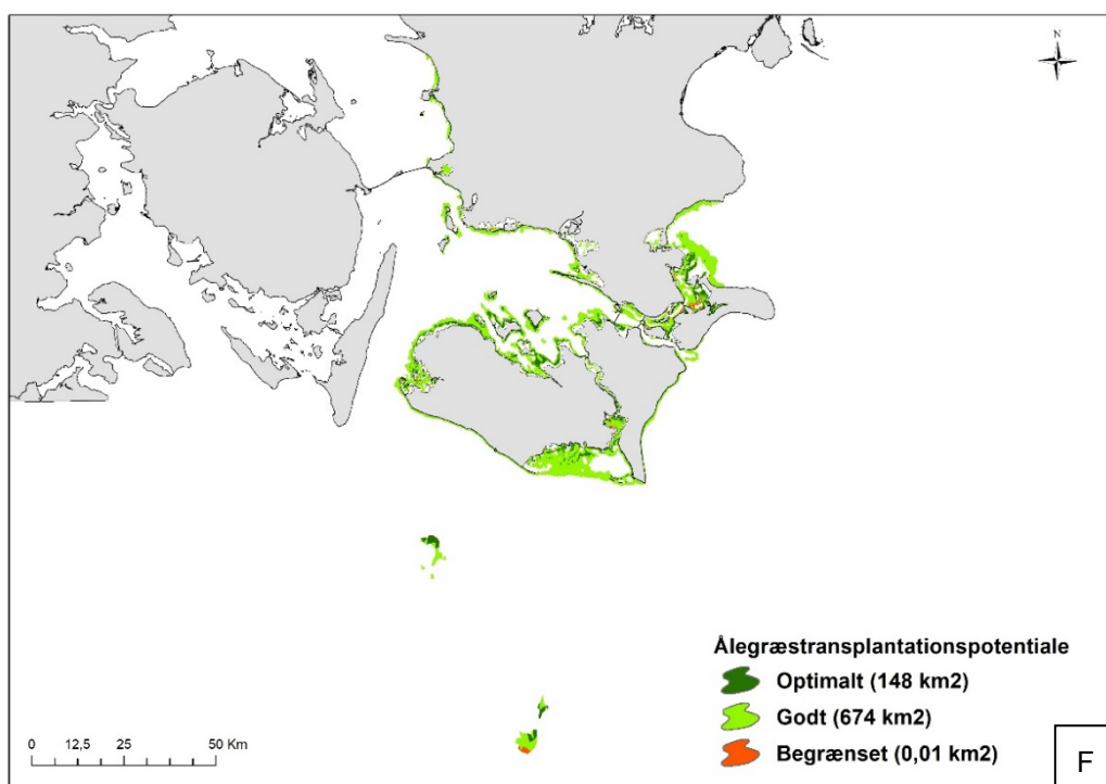
Figur 4.1. Potentialer for ålegræstransplantering (bruttoareal) i udvalgte vandområder fastlagt med GIS model og modelgenererede datalag for lys, frekvens af resuspension, iltforhold, bundforhold, ballistiske påvirkninger fra makroalger og DIN koncentration. Datalag er genereret ud fra DHI's Vandplanssimuleringsresultater. A, Limfjorden model. B, Mariager Fjord model. C, NBF model. D, Odense Fjord model. E, Roskilde Fjord model. F, Smålandsfarvandet model. Bemærk at Isefjorden ikke er analyseret. Grøn markering angiver områder med potentiale for transplantering og rød angiver områder, hvor lysforholdene er på grænsen til at kunne understøtte transplantering. Oversigt over vandområder, som indgår i analysen kan ses i appendix B.
