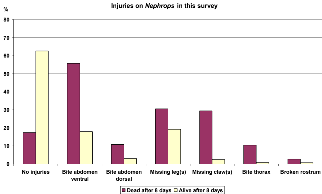
Fig. 30. Resultater af undersøgelse af 1744 jomfruhummere for skader.
