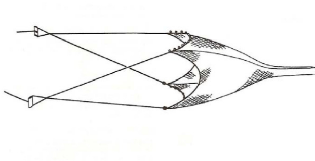
Figur 4.3.6. Pelagisk trawltype til bundnært fiskeri efter tobis, sild og brisling. Se FAO(2014).
