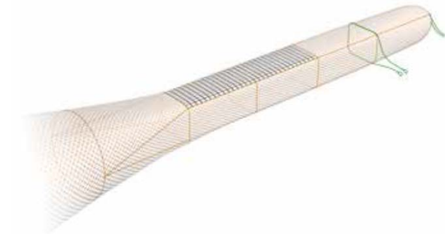
Figur 4.2.3.1. Skematisk fremstilling af en SELTRA fangstpose. Bemærk at fangstposen er opbygget i 4 lige paneler hvor selektionsvinduet er placeret i sektionens øvre side. Denne 4-panel fangstpose kan monteres både med og uden kiler til redskabets 2-panel design. På figuren er markeret en kort kile i denne overgang. Figuren er gengivet med tilladelse fra SEAFISH.
