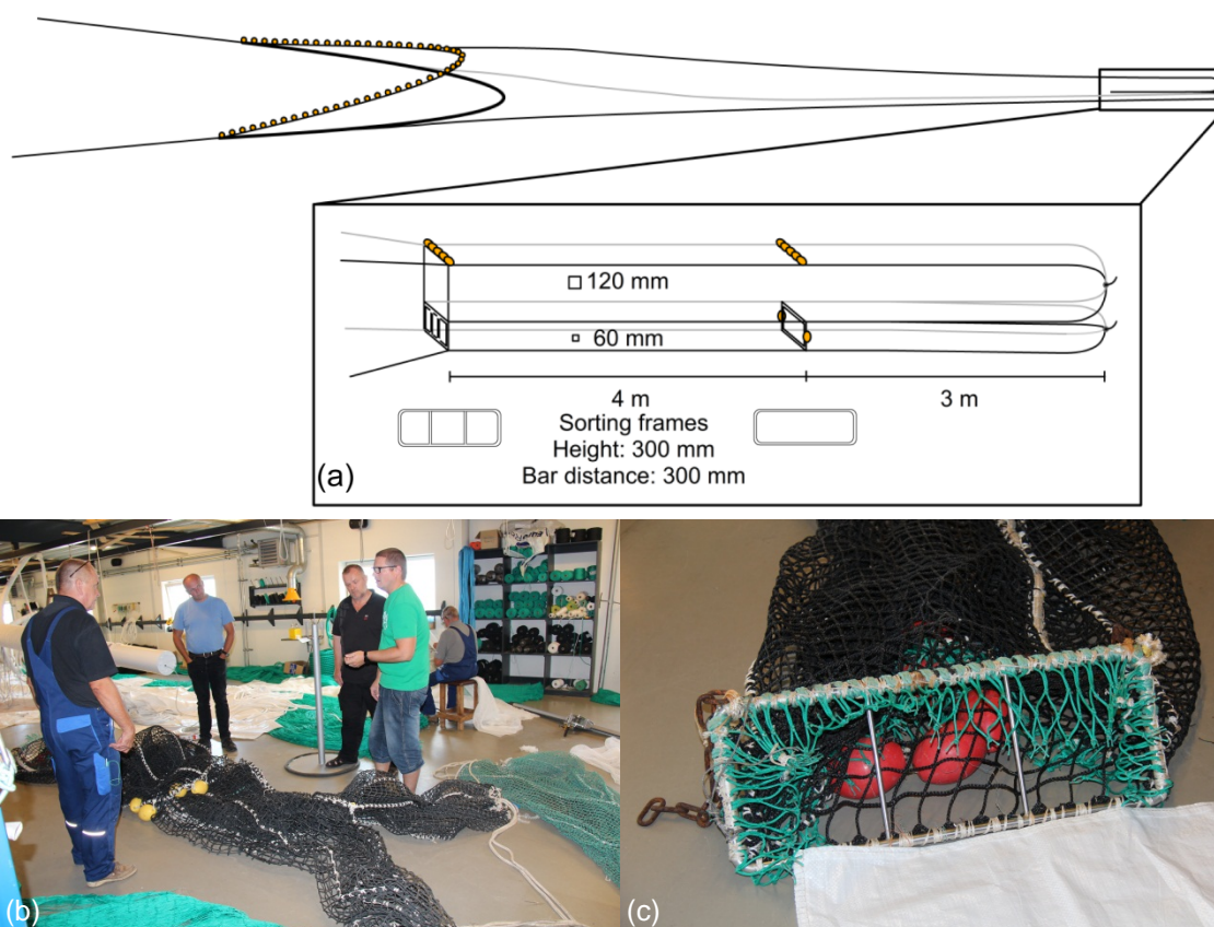
Fig. 4.4.1.1. Den horisontaldelte fangstpose. Skematisk illustration (a). Udvikling og produktion i samarbejde med vodbinder og fiskeskipper (b). Sorteringsramme der var monteret i skæringen mellem trawlstykket og fangstposen (c).
