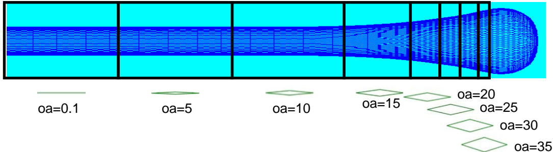
Fig. 4.1.1.1. Simulerede maskeåbninger i en diamantmaskepose lavet af 4 mm dobbelt-tråd, med 100 masker rundt og en fangstvægt på 100 kg. Det ses at åbningsgraden (oa) er størst umiddelbart foran fangsten. Figuren er lavet ved hjælp af simuleringværktøjet PRESEMO der er beskrevet i Herrmann, B. (2005) Effect of catch size and shape on the selectivity of diamond mesh cod-ends. I. Model development. Fisheries Research, 74, 243-252.
