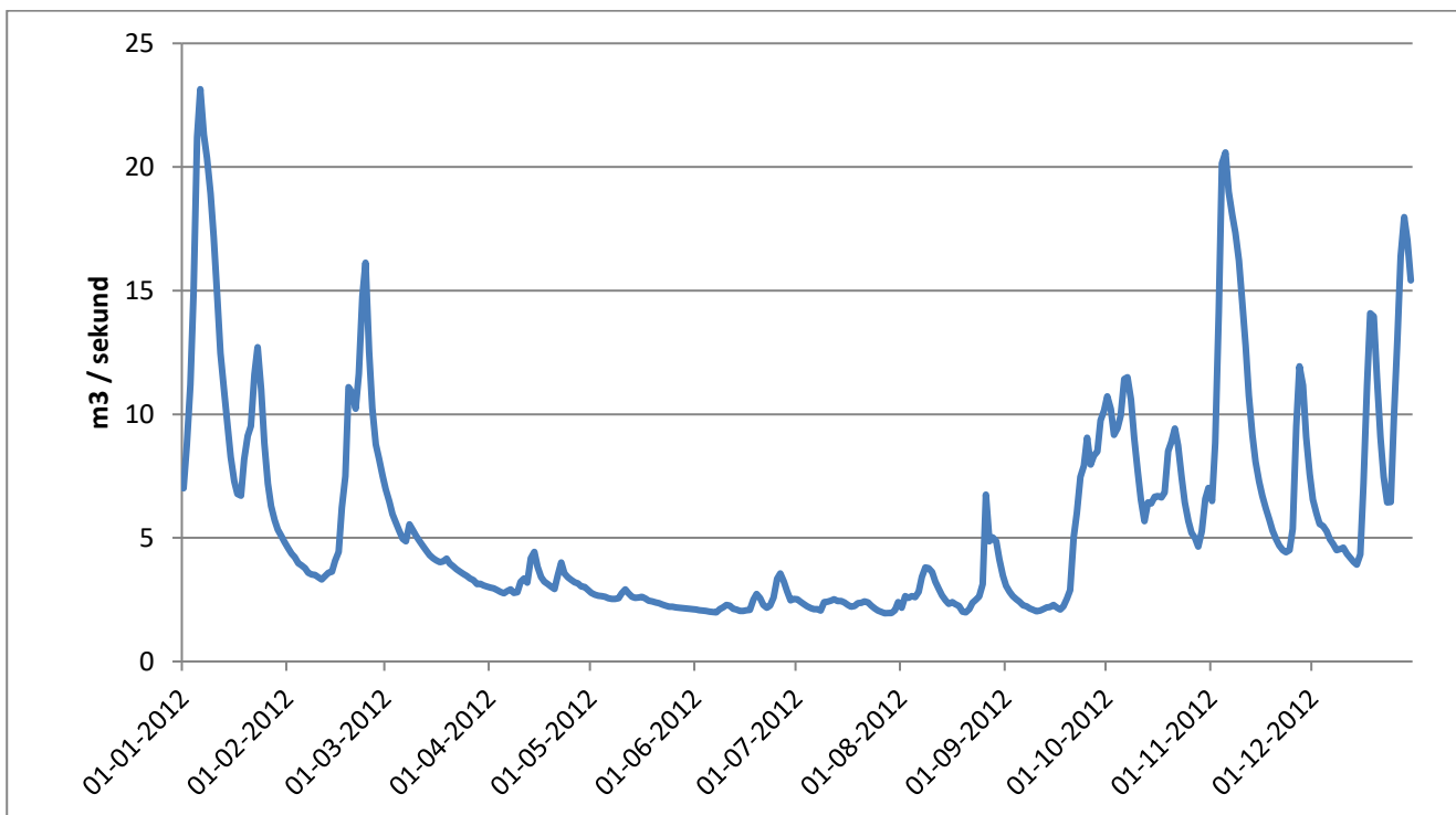
Figur 6: Vandføringen i 2012.
