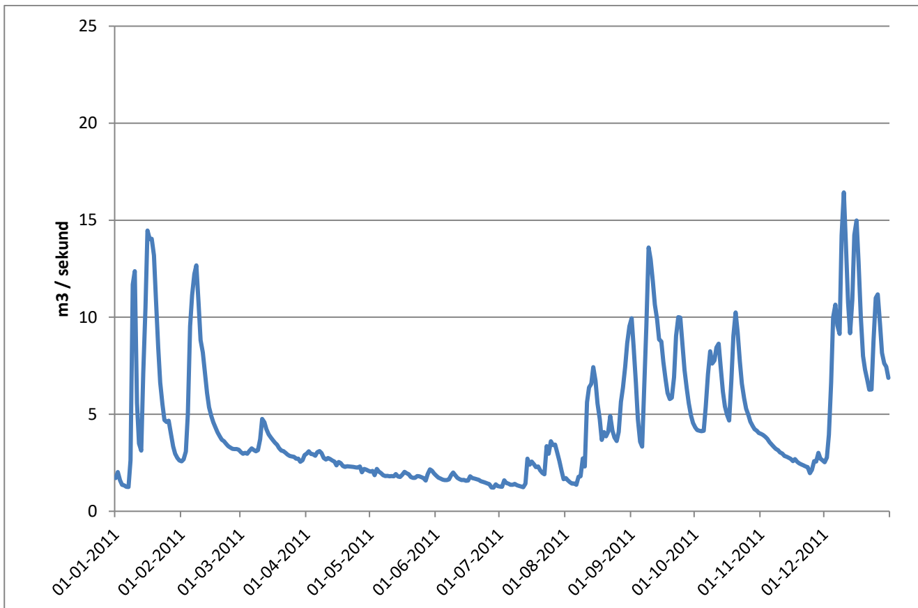
Figur 5: Vandføringen i 2011.
