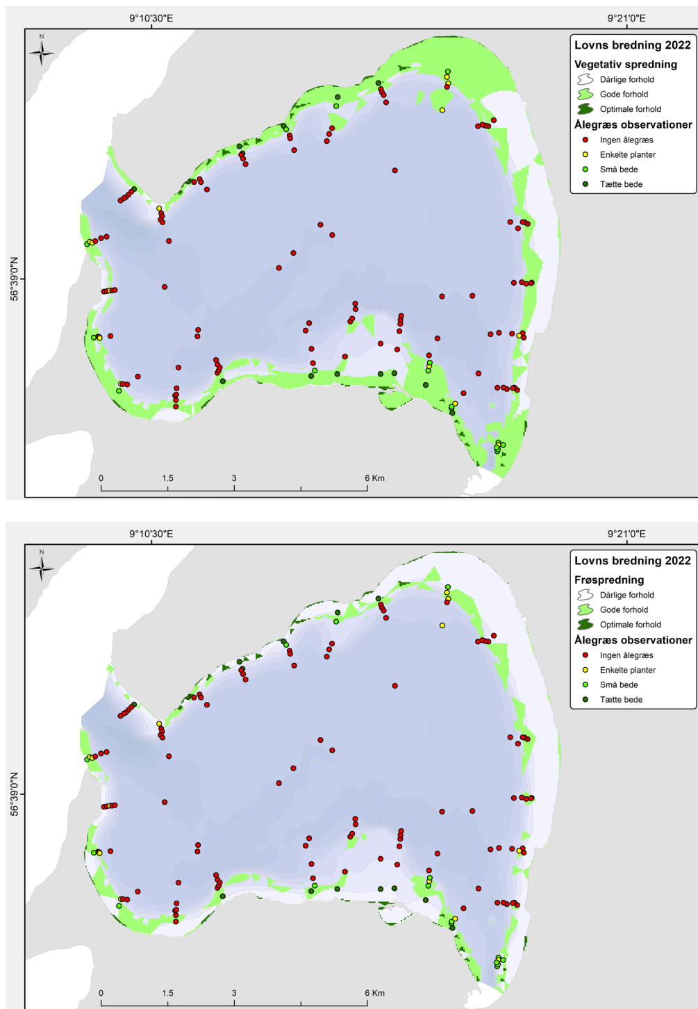
Figur 7. Modellering af ålegræssets mulighed for re-kolonisering i Lovns Bredning ved henholdsvis vegetativ spredning (øverst) og ved frøspredning (nederst). Modellen er baseret på i alt ni miljøparametre, der er udslagsgivende for ålegræssets etablering. Mørkegrønne og lysegrønne områder markerer områder, der er henholdsvis optimale og gode for ålegræssets etablering. Punkter indikerer de reelle observationer i maj 2022.
